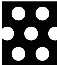
15 8φ×13P 開孔率(約34%)
