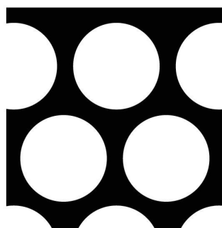
18 15φ×20P 開孔率(約51%)
