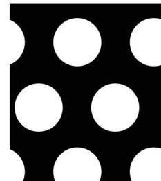
16 10φ×15P 開孔率(約40%)
