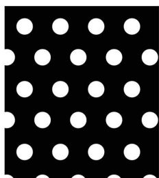
9 4φ×7P 開孔率(約30%)
