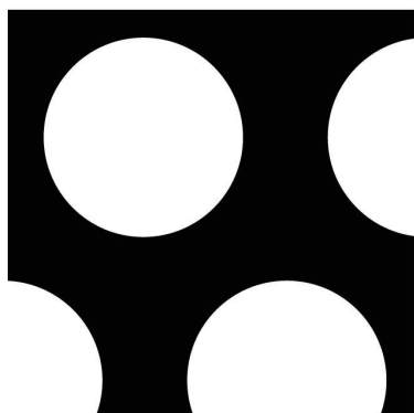
20 25φ×35P 開孔率(約46%)
