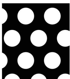
14 8φ×12P 開孔率(約40%)
