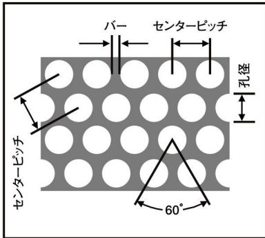
丸孔60°千鳥
