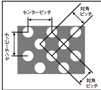
丸孔角千鳥(45°)
